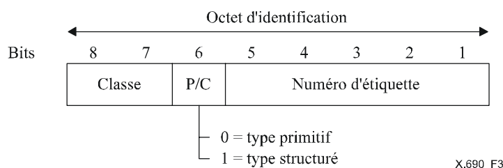
Figure 3 – Champ d'identification à un octet (étiquette de petit numéro)
