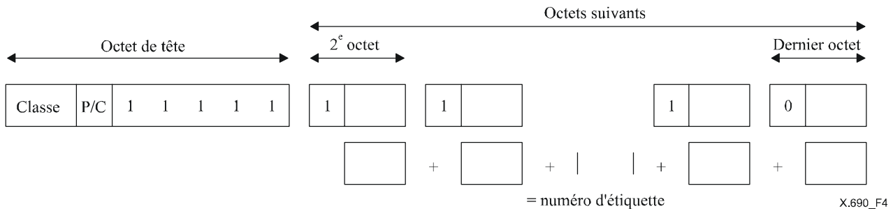
Figure 4 – Champ d'identification à plusieurs octets (étiquette de numéro élevé)
