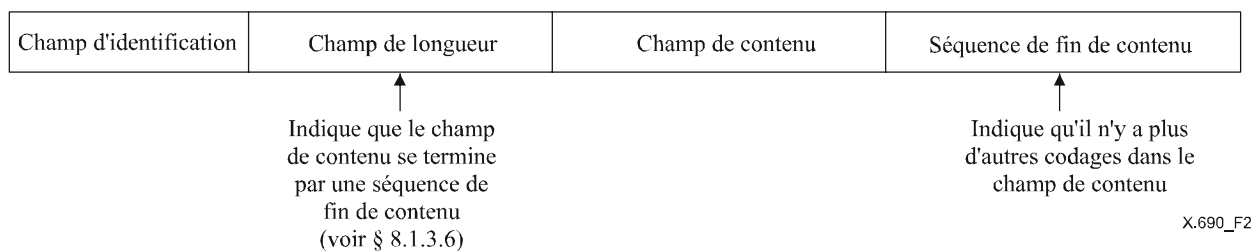
Figure 2 – Variante de codage structuré
