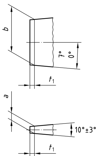
Figure 1 — Modèle A, pour tournevis à main seulement
