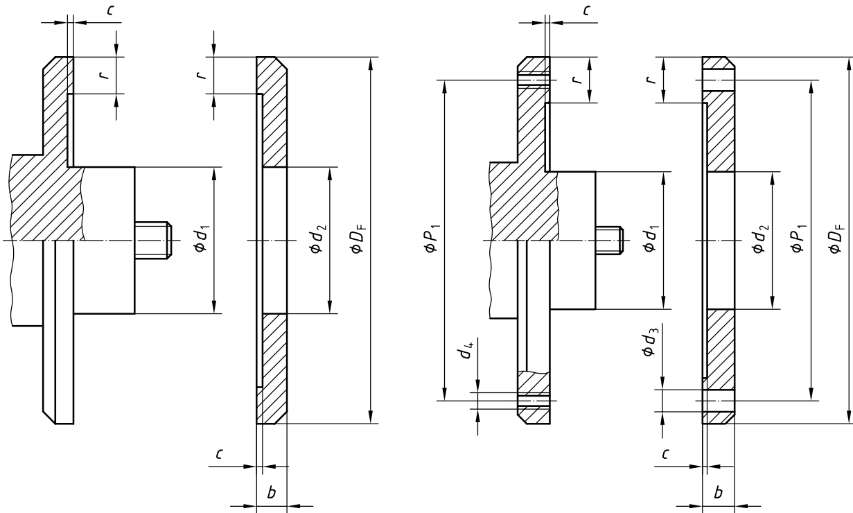
Figure 1 — Type N1 sans trou d'ergot
