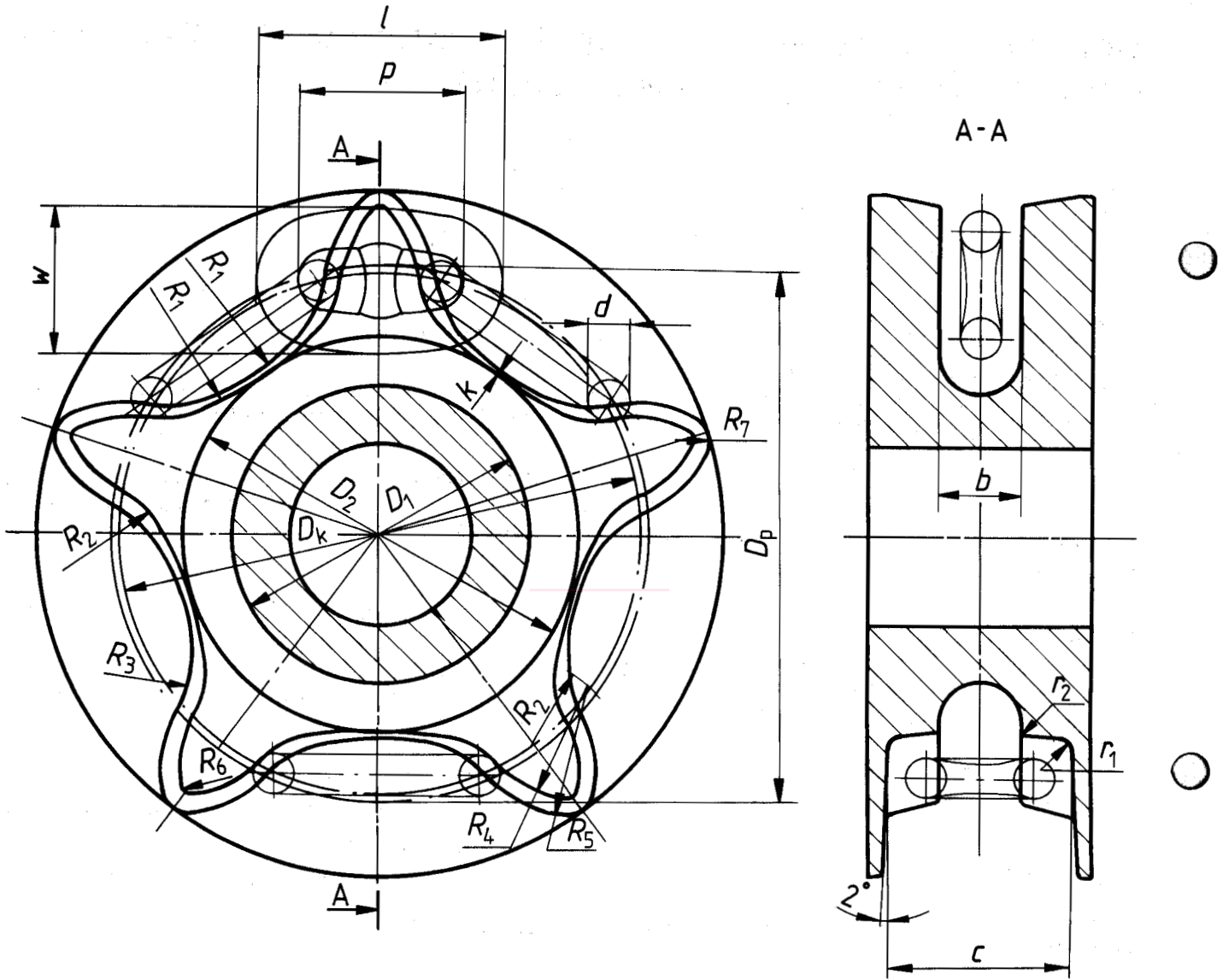
Figure — Barbotin pour les chaînes d'ancre étançonnées
