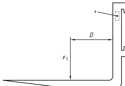
Figure 1 — Emplacement du marquage et position d'application des charges d'épreuve
