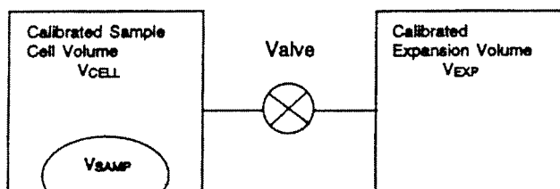
FIG. 2 Pycnometer Apparatus
