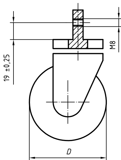
Figure 3 — Roulette à tige pleine avec trou de fixation taraudé
