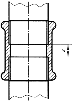
Figure 3 — Longueur de pose z dans le cas d'un raccord droit
