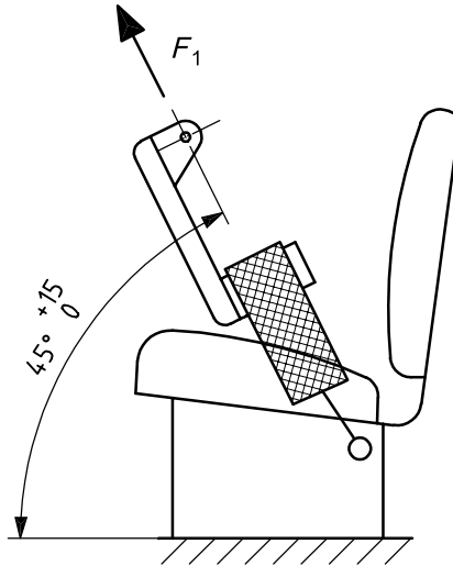
iTeh STANDARD PREVIEW Figure 4 — Essai de traction vers l'avant — Application de la force (standards.iteh.ai)
