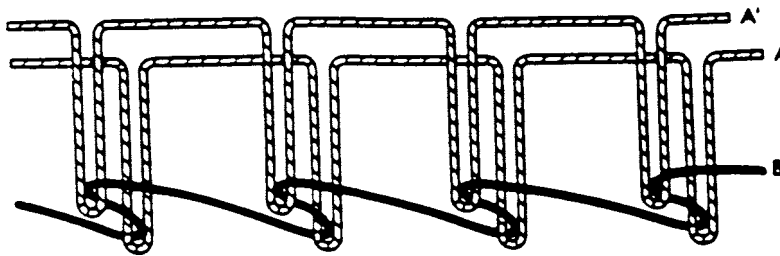
FIG. 19 Stitch Type 309
