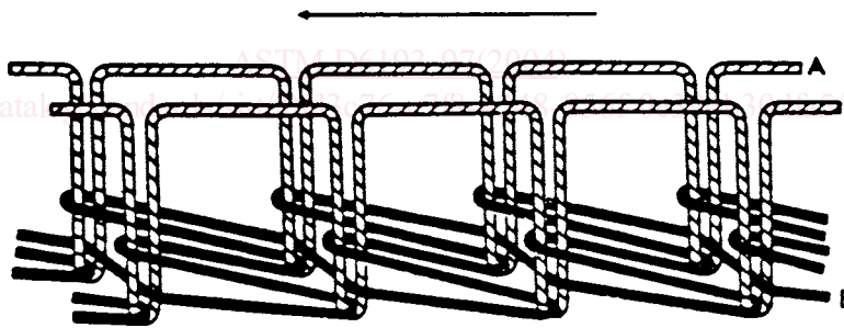
FIG. 31 Stitch Type 405
