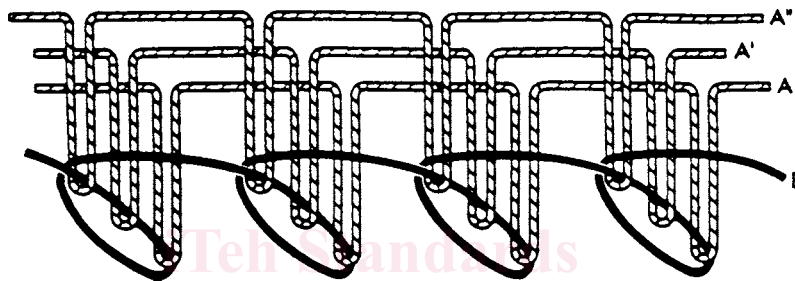
FIG. 13 Stitch Type 303
