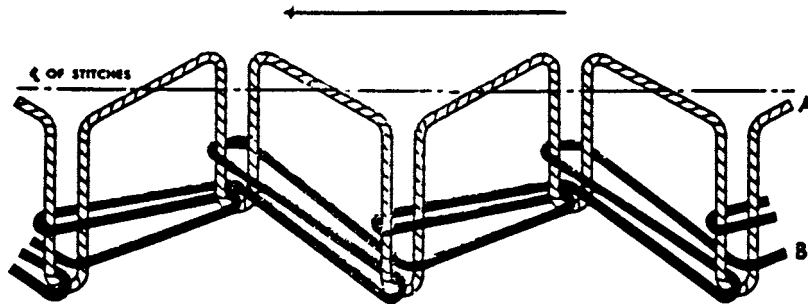
FIG. 30 Stitch Type 404
