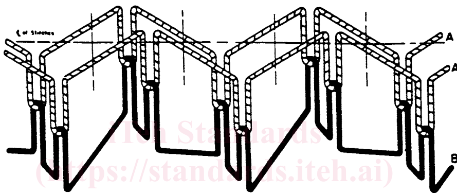
FIG. 22 Stitch Type 312
