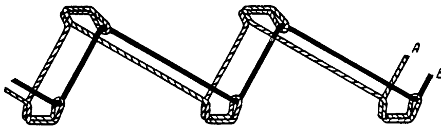
FIG. 23 Stitch Type 313
