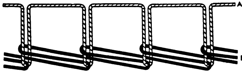
FIG. 27 Stitch Type 401
