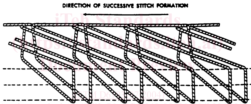
FIG. 33 Stitch Type 407
