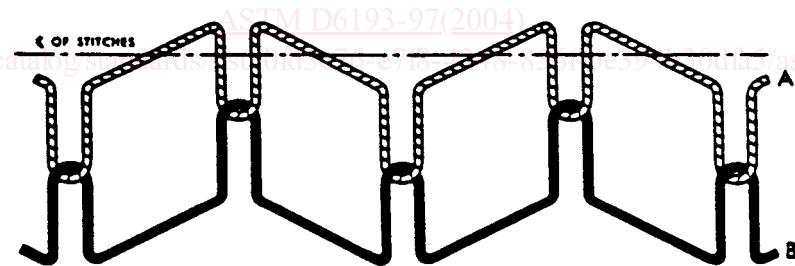
FIG. 14 Stitch Type 304
