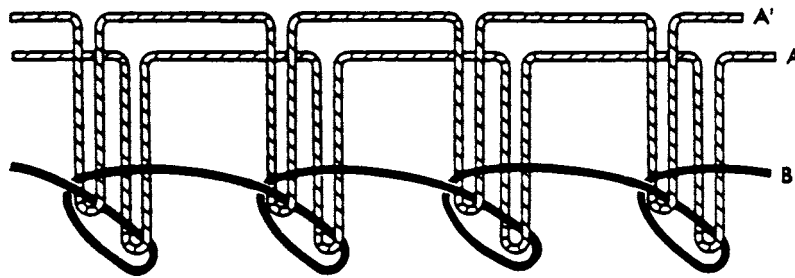
FIG. 12 Stitch Type 302
