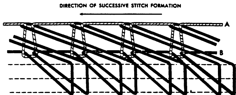
FIG. 34 Stitch Type 501
