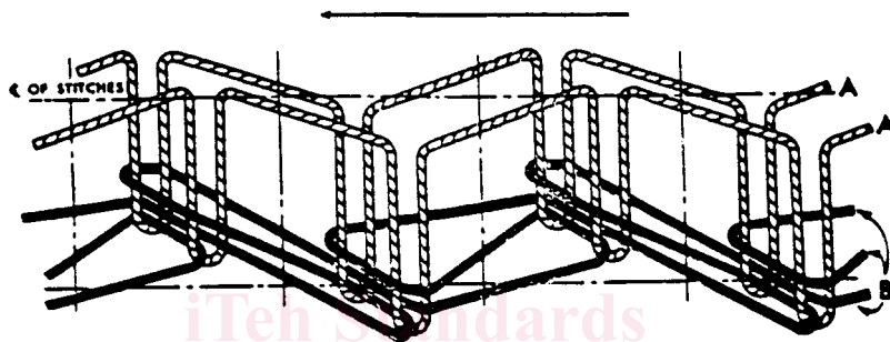
FIG. 31 Stitch Type 405
