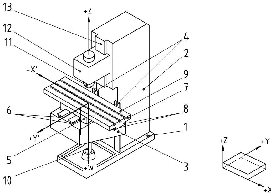
Figure 1 — Machines à fraiser à table à hauteur variable, à broche verticale et à tête porte-broche coulissant verticalement
