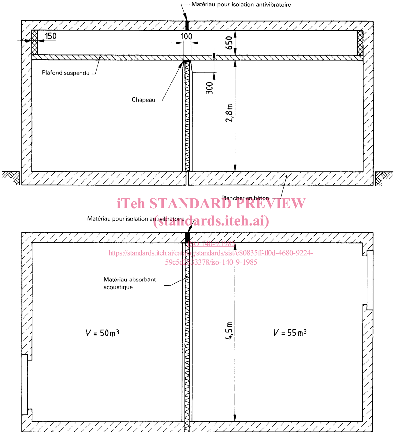
Figure — Coupe transversale et plan de l'installation d'essai (Les dimensions sont données à titre indicatif; des spécifications générales sont donnés au chapitre 5.)
