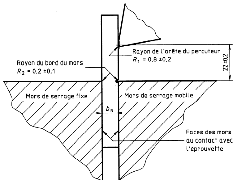
Figure 2 — Support d'éprouvette et arête du percuteur représentés à l'impact de l'éprouvette entaillée
