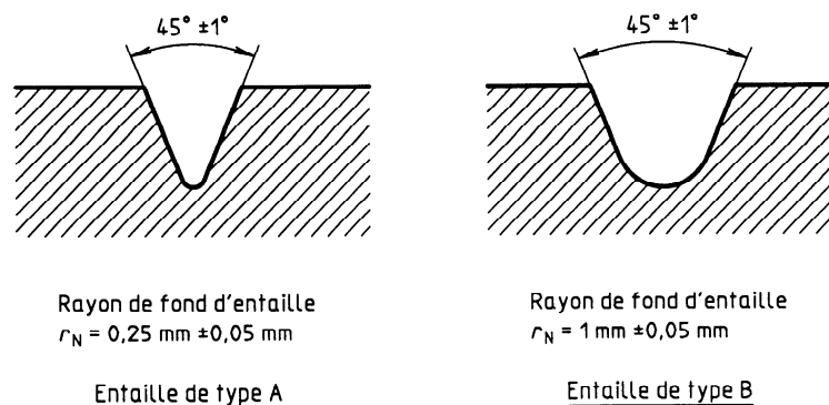
Figure 3 — Types d'entailles
