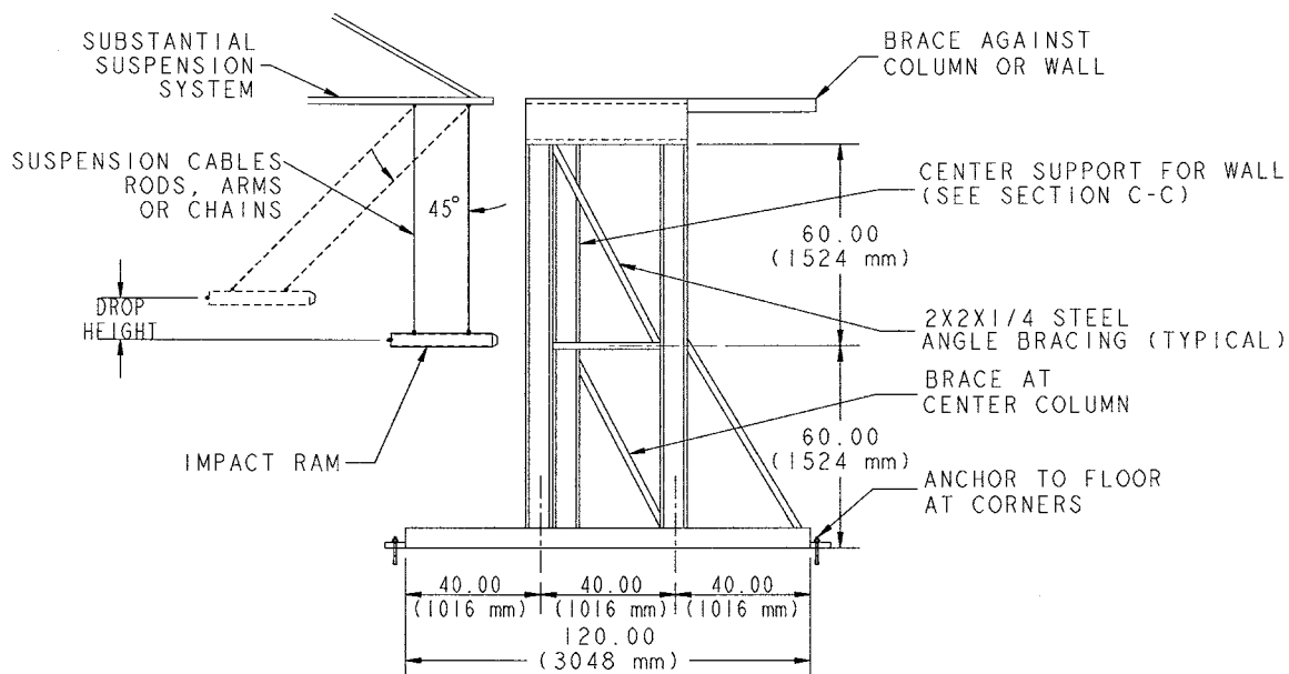
FIG. 2 Test Wall
