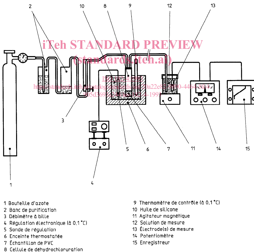
Figure 1 — Disposition générale de l'appareillage
