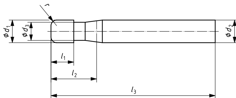
Figure 1 — Type 1: Fraises toriques deux tailles, courtes
