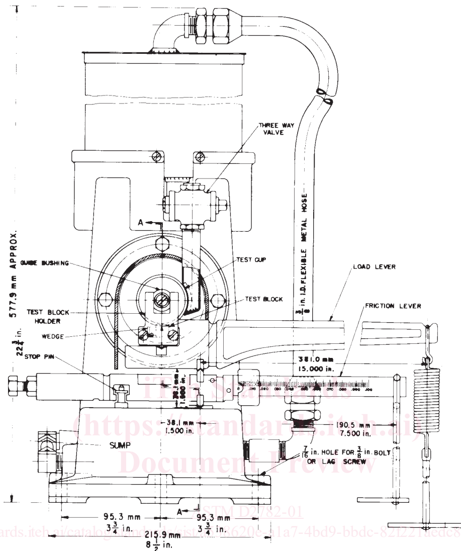
FIG. 2 Timken Tester
