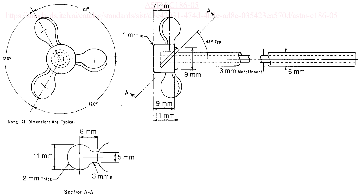
FIG. 2 Stirrer
