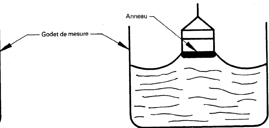
Figure 5 – Anneau comme corps de mesure
