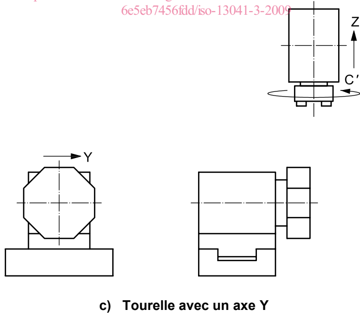
Figure 1 — Trois configurations de machine avec un porte-pièce et une tourelle
