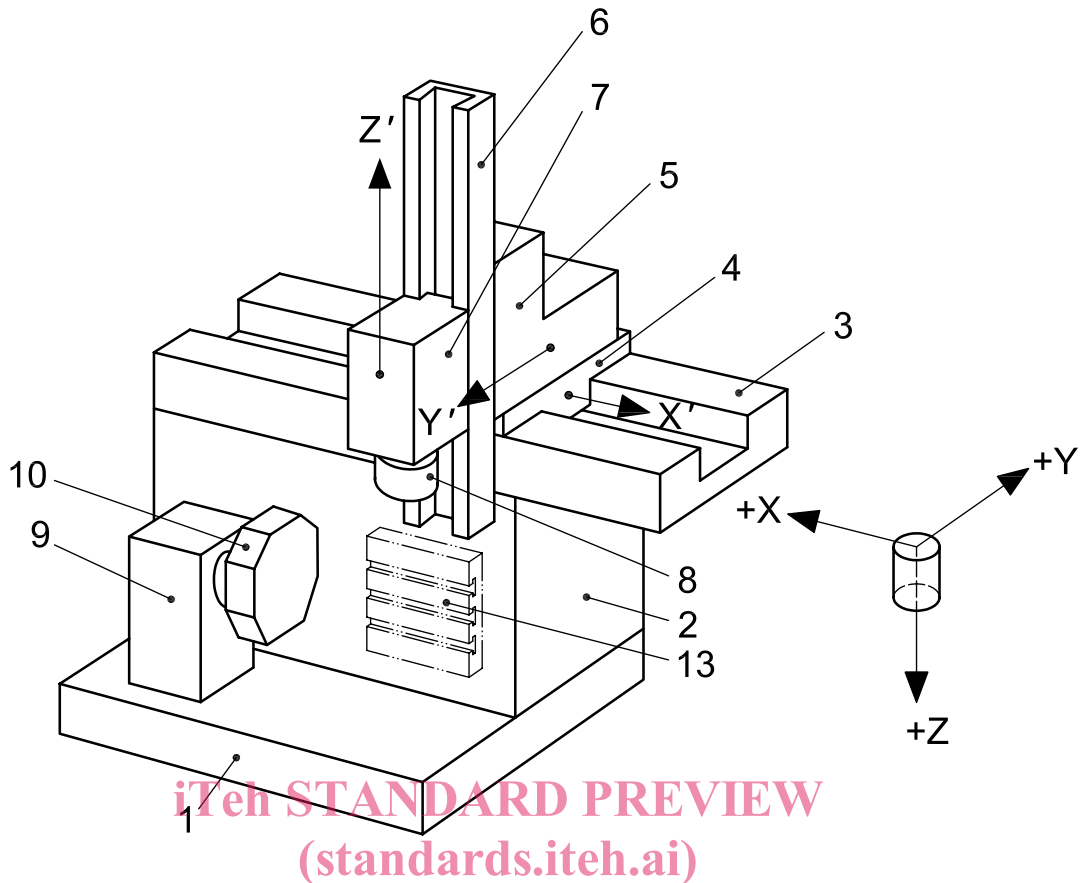
Figure 4 — Exemple de centre de tournage à broche verticale inversée (broche avec un mouvement sur l'axe Y)
