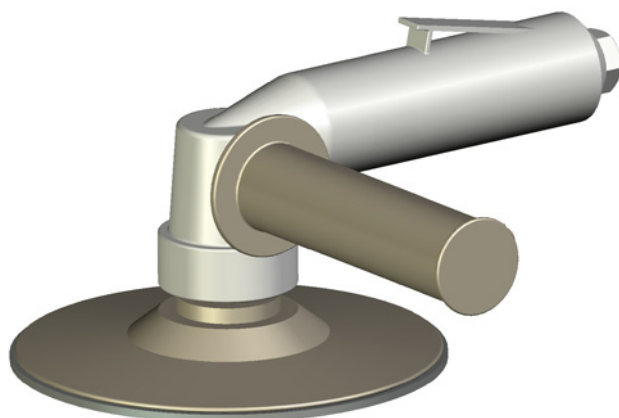
Figure 2 — Ponceuse rotative d'angles/Polisseuse-lustreuse sur laquelle le moteur sert de poignée principale
