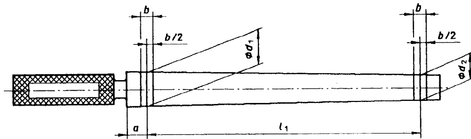
Figure 3 — Calibre pour tubes type A
