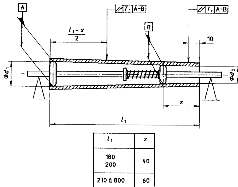
Figure 2 — Mesurage du battement total, T_r
