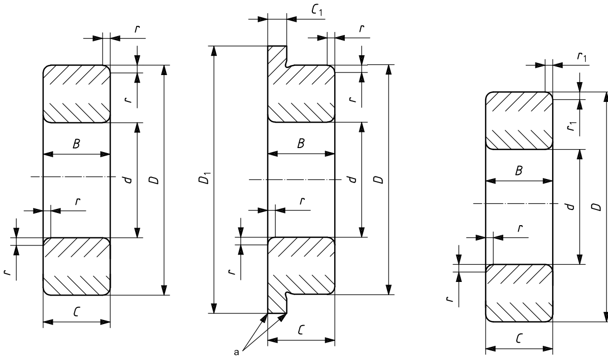
a) Roulements à billes à une rangée à gorge profonde
