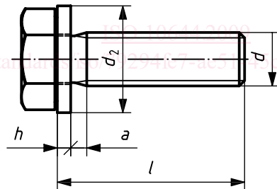
Figure 1 — Vis filetée jusque sous la rondelle
