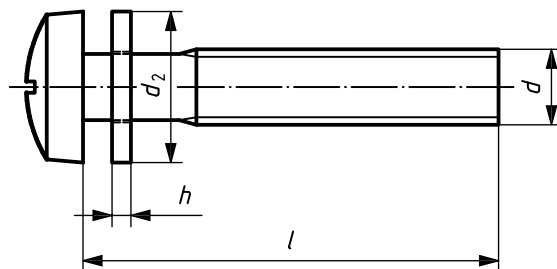
Figure 1 — Vis filetée jusque sous la rondelle
