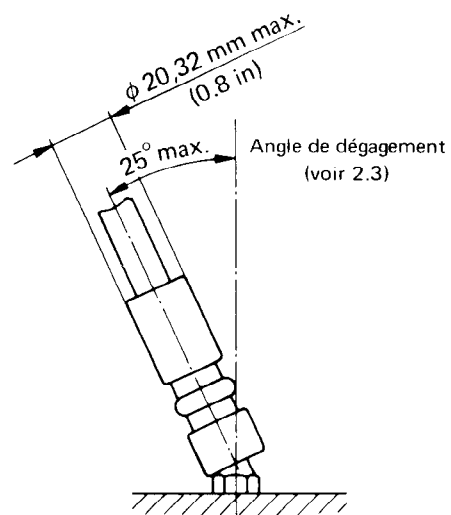
FIGURE 2 — Aagrafe de la pompe de graissage — Conditions d'accrochage et de décrochage
