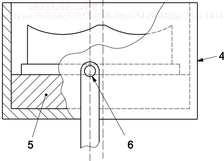
Рисунок 2 — Конфигурация испытательного образца
