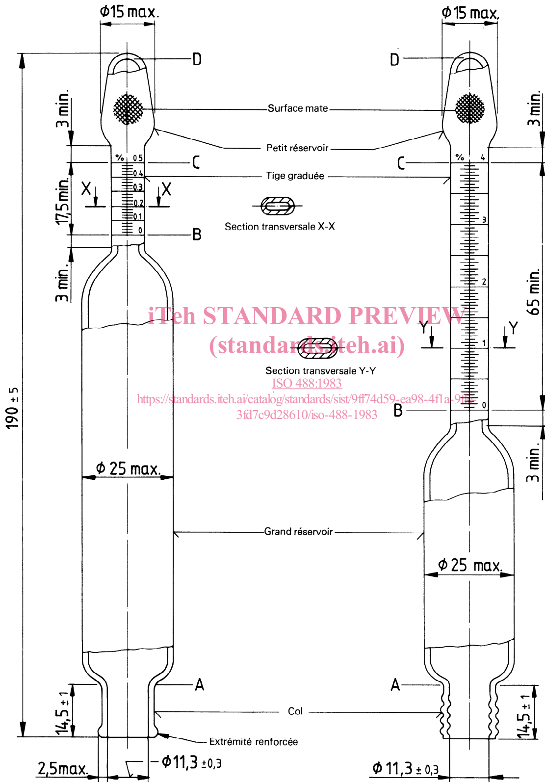
Figure 1 — Butyromètre de 0 à 0,5 %, à col lisse
