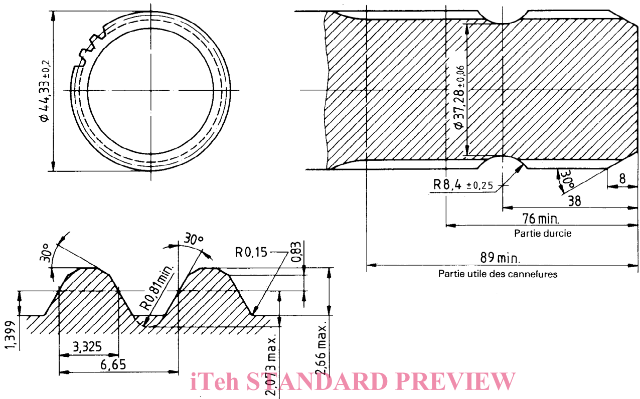
Profil de base de l'arbre
