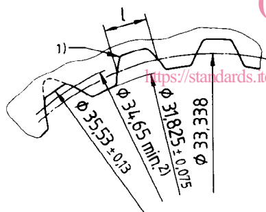
Profil du moyeu
