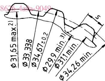
Profil de l'arbre
