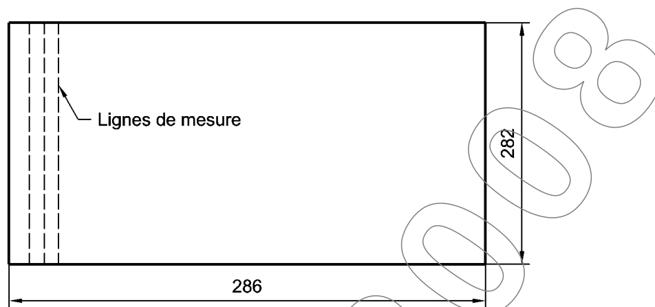
Figure B.2 — Zone de mesure de l'étalon de régularité d'aspect
