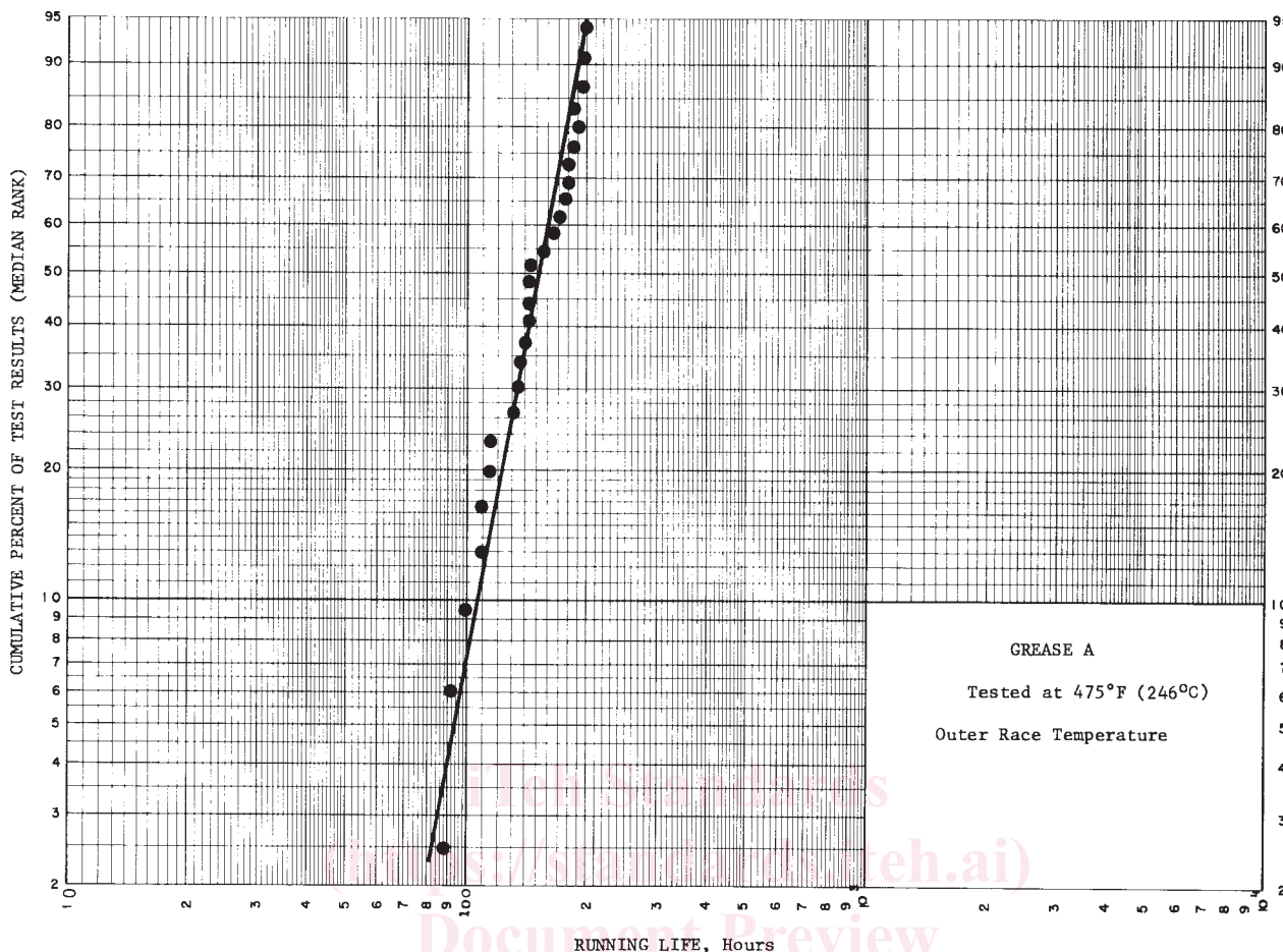
FIG. 1 Weibull Parameter of Grease A
