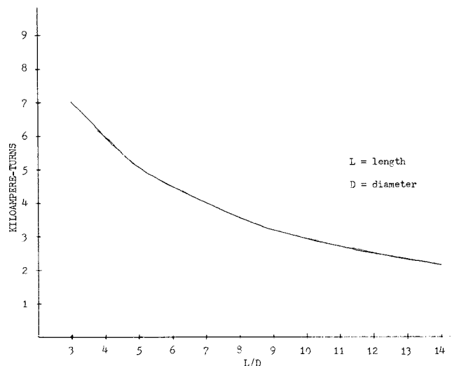
FIG. 7 Longitudinal Magnetization
