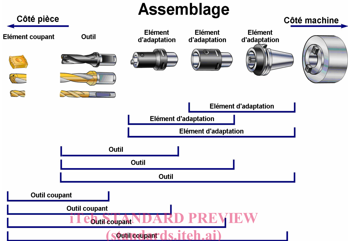
ISO/TS 13399-150:2008 https://standards.iteh.ai/catalog/standards/sist/c057f5f8-3401-4e60-a6cc-1d14c2771525/iso-ts-13399-150-2008 Figure 1 — Assemblages de différents types d'éléments
