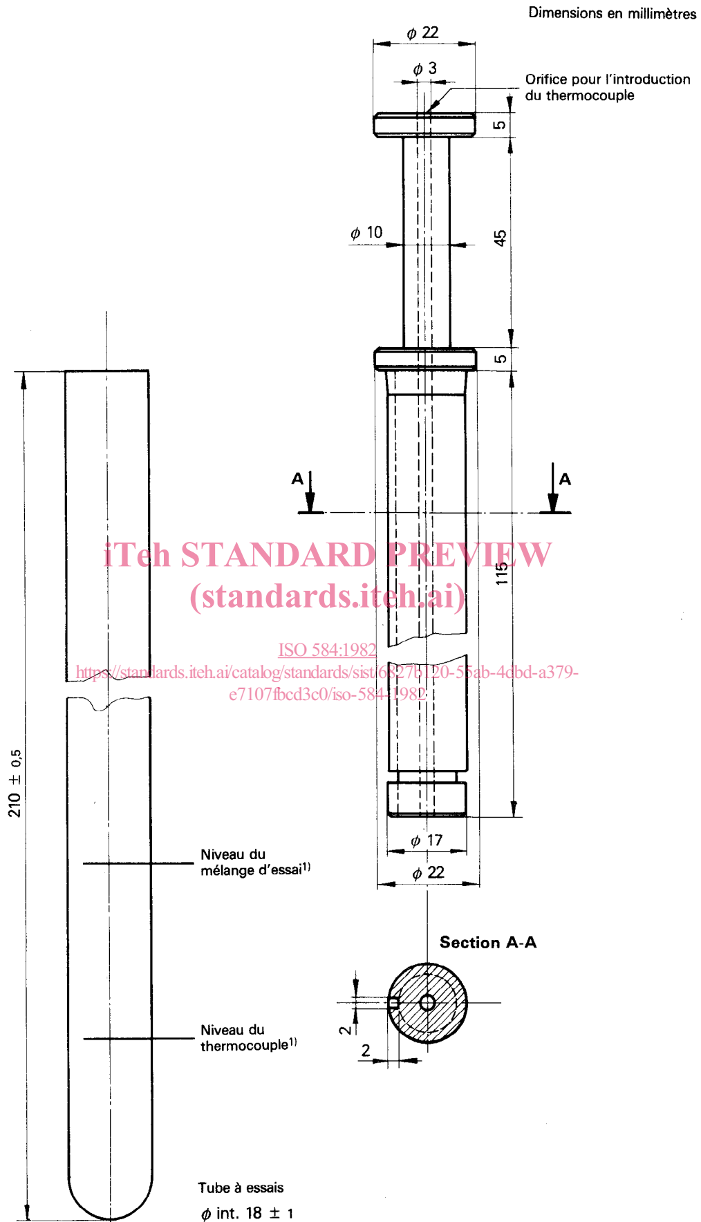
Figure — Exemple de dispositif de centrage du thermocouple
