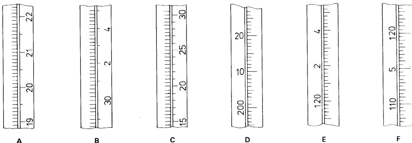
Figure 2 — Différents types de graduation et de chiffrage
