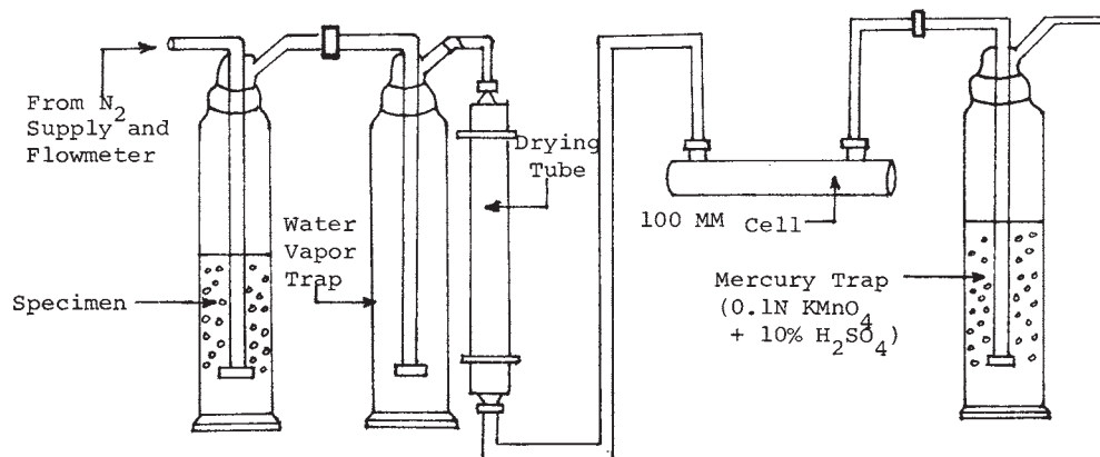
FIG. 1 Apparatus
