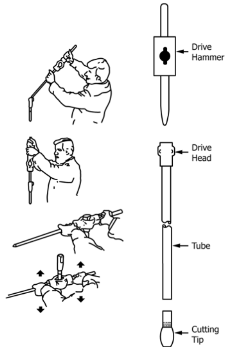
FIG. 7 Veihmeyer Tube
