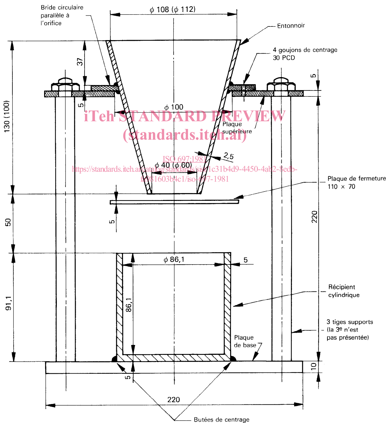
Figure — Appareillage pour la détermination de la masse volumique apparente des poudres ou granulés
