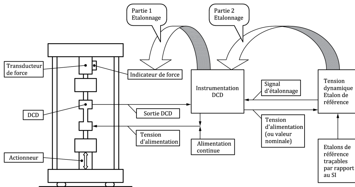
Figure 1 — Schéma de la méthodologie d'étalonnage ISO 4965 (transducteur → Cellule,)
