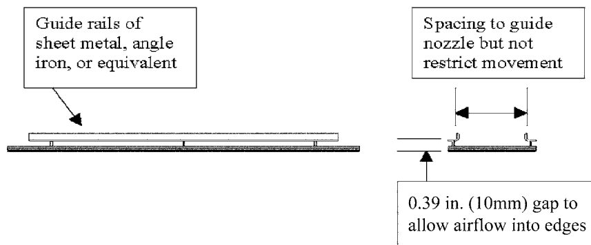
FIG. 1 Guide Rails
