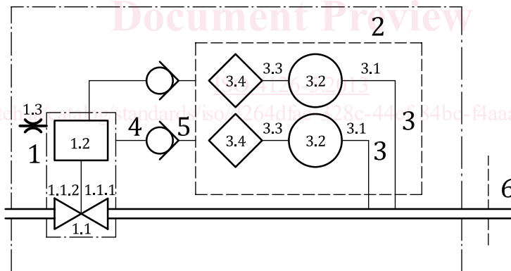
b) Une ligne de commande, principe de décharge
