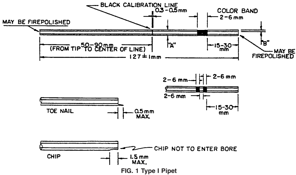
FIG. 1 Type I Pipet
