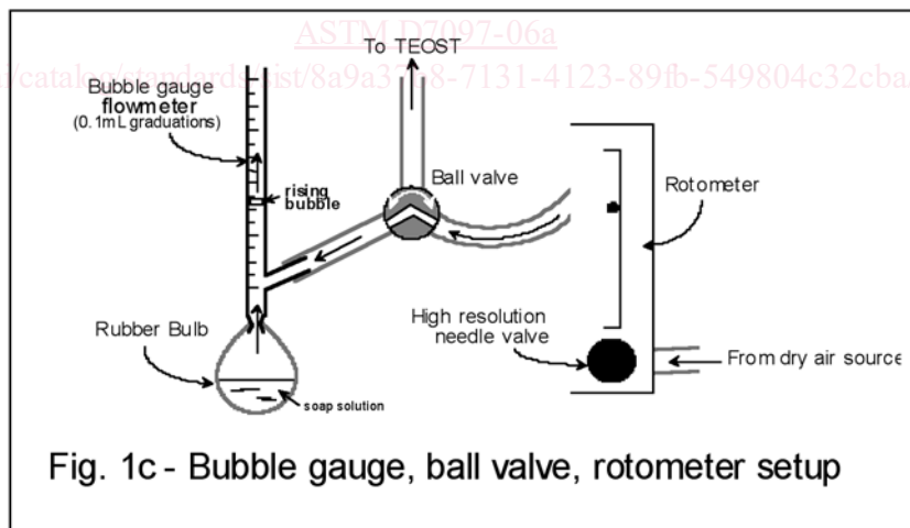
FIG. 1 Bubble Gage
