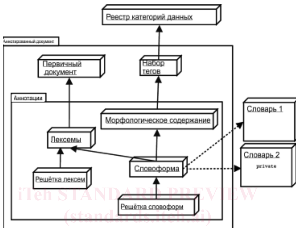
Рисунок 1 — Упрощённый вид метамодели MAF
