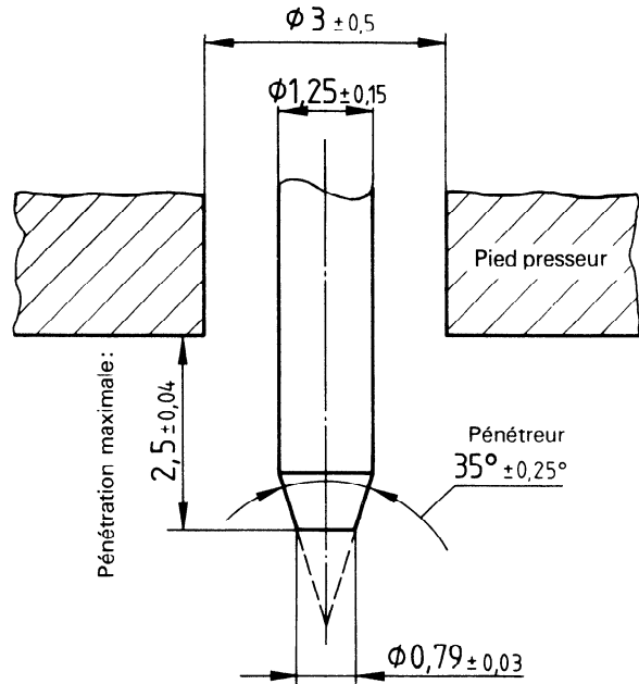
Figure 1 — Pénétreur pour le duromètre du type A
