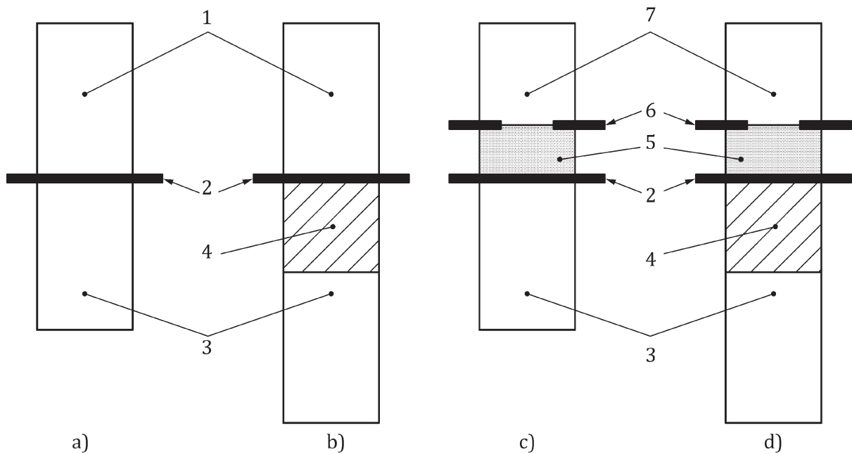
a) Interface directe b) Interface de support intermédiaire c) Interface directe (quand combinaison d'un actionneur multitours et d'un réducteur multitours/linéaire) d) Interface de support intermédiaire (quand combinaison d'un actionneur multitours et d'un réducteur multitours/linéaire)
