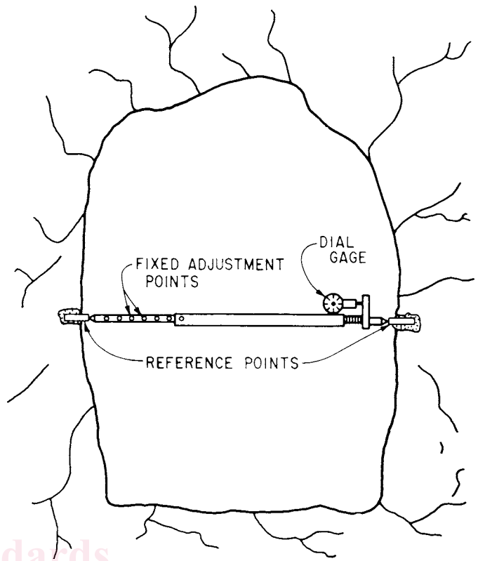
FIG. 2 Bar Extensometer
