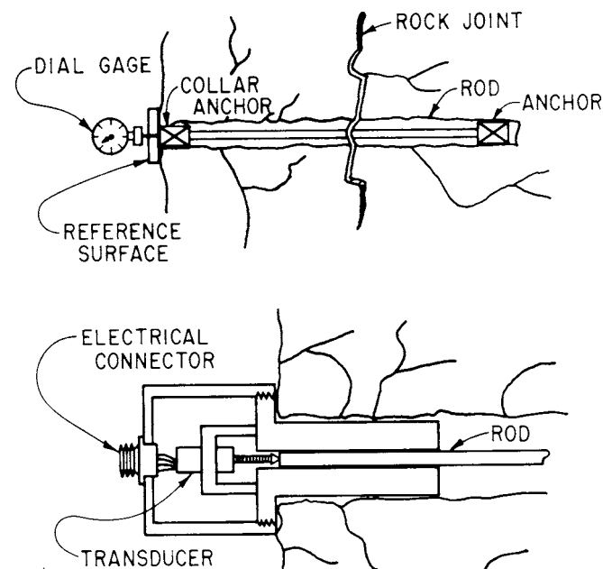
FIG. 1 Rod Extensometer
