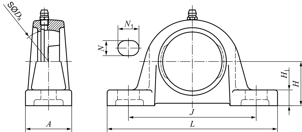
Figure 1 — Corps de palier à semelle moulé
