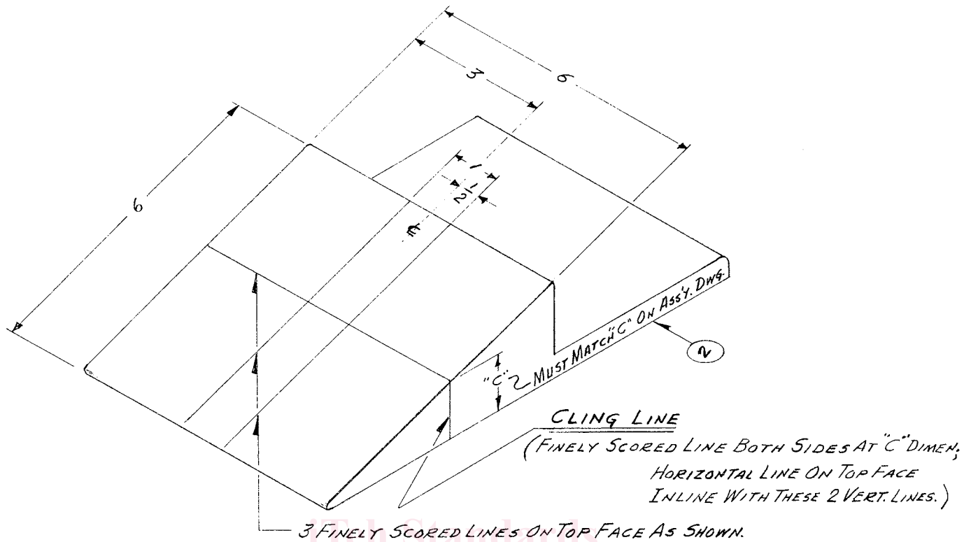
FIG. 2 Incline Surface
