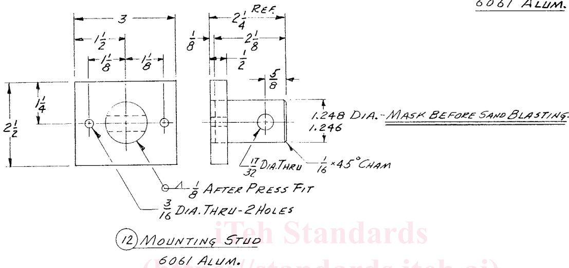
FIG. 3 Mounting Stud
