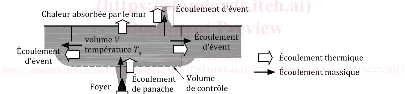
Figure 1 — Conservation générale de la chaleur et de la masse dans une enceinte en présence d'une source de feu
