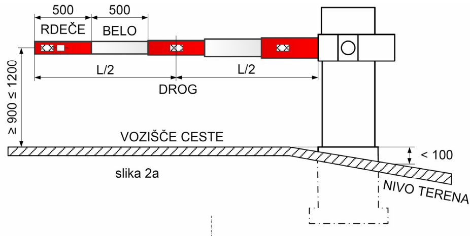
Slika 1: Shematski prikaz (pol)zapornice
